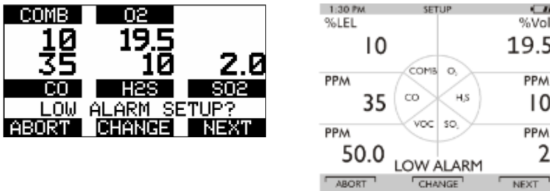
Figura 13 Configuração de Alarme de Sensor
