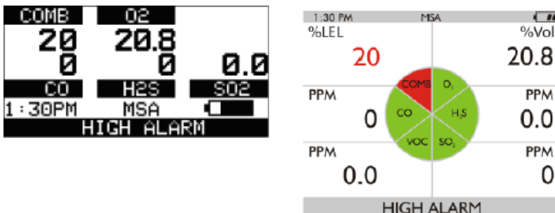
Figura 9 Condições de alarme (aqui Alarme Alto)
