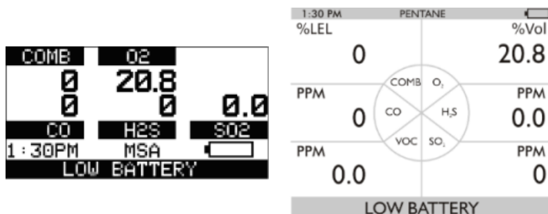
Figura 5 Advertência de bateria
